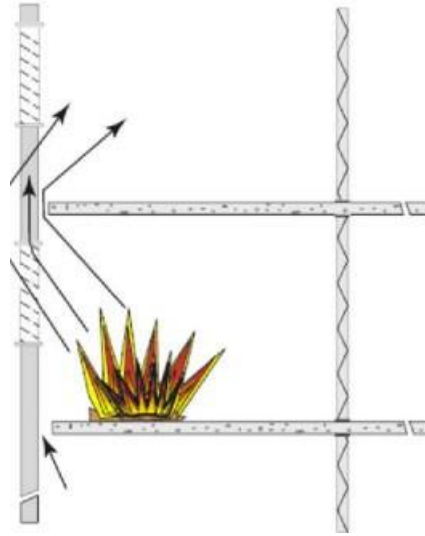
Şekil 18. Bir Katmanlı Olan Cephede Yangın Yayılımı
