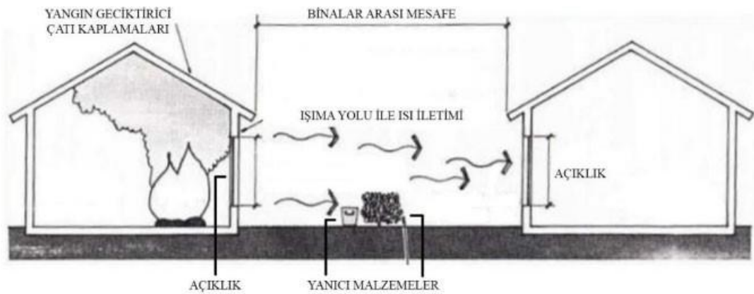
Şekil 20. Işıma Yolu ile Yangının Binalar Arası Yayılması
