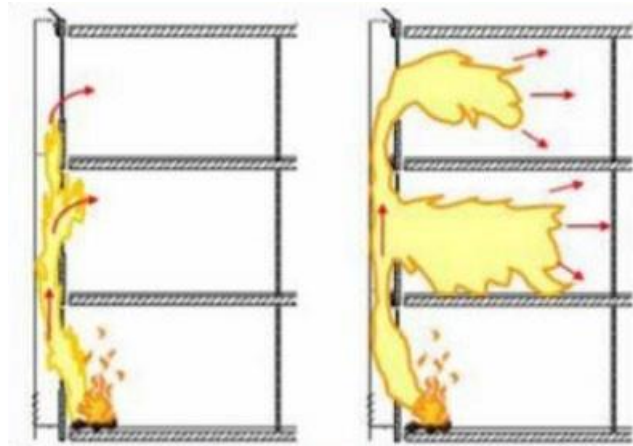
Şekil 19. Çift Katmanlı Cephede Yangın Yayılımı
