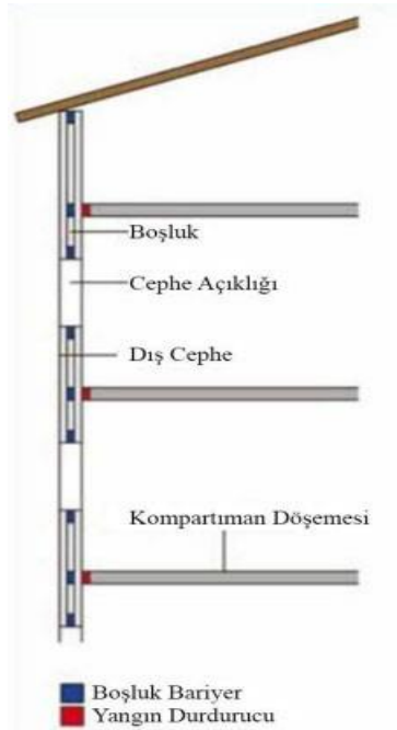
Şekil 17. Boşluk Bariyerlerinin Düzenlenmesi
