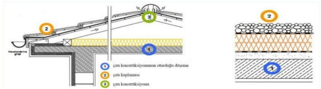
Şekil 15. Çatı Malzeme Detayı
