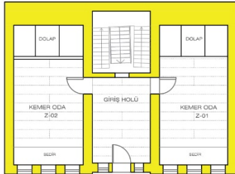
ZEMİN KAT PLANI
