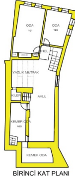
BİRİNCİ KAT PLANI
