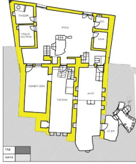
ZEMİN KAT PLANI
