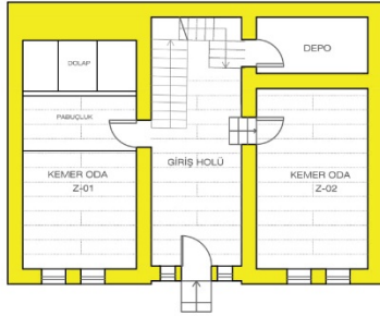
ZEMİN KAT PLANI
