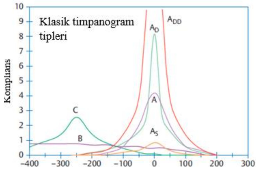
Şekil 6. Timpanogram tipleri (Gelfand, 2016).
