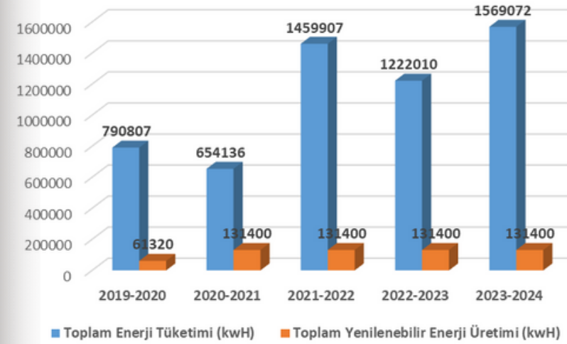
2019-2024 Yılları Arası Yıllık Enerji Tüketimi ve Yenilenebilir Enerji Üretimi Miktarları
