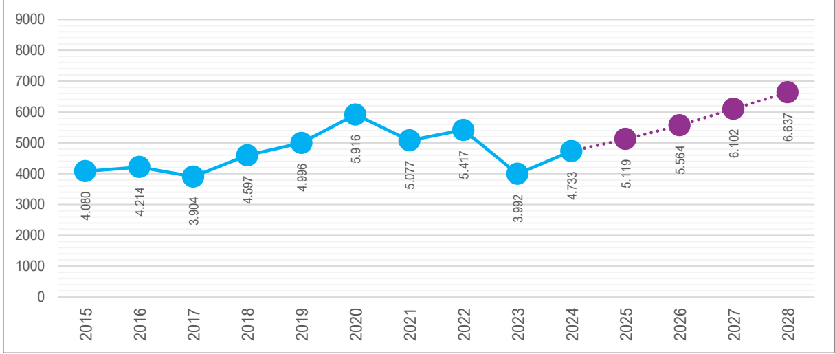
Şekil 4.3.1. Artvin'in yatak kapasitesi ve tahminler
